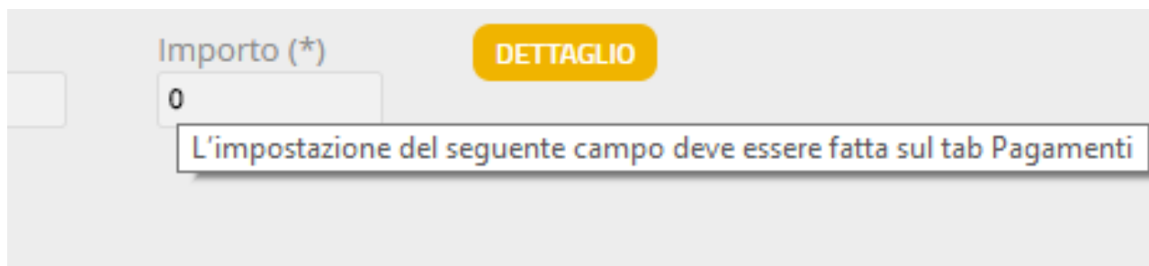
Figura 8: Tooltip sull'importo
